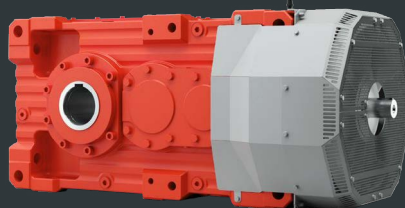
Réducteurs industriels
